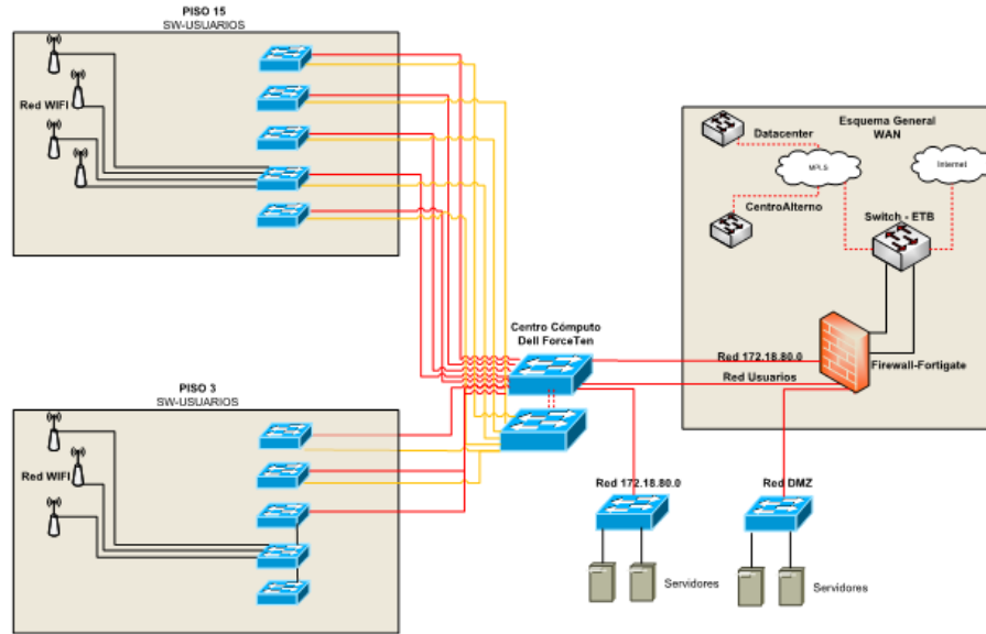
Ilustración 3 Topología de la red de comunicaciones
